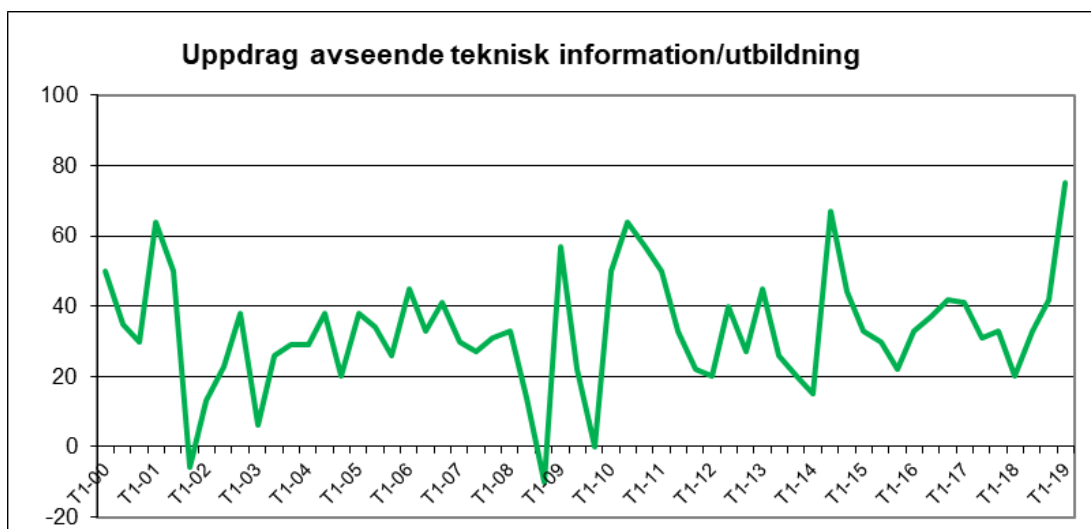
Diagram 16: Industrikonstulernas förväntningar på orderstockens utveckling för uppdrag avseende teknisk information/utbildning. Netttotal.
