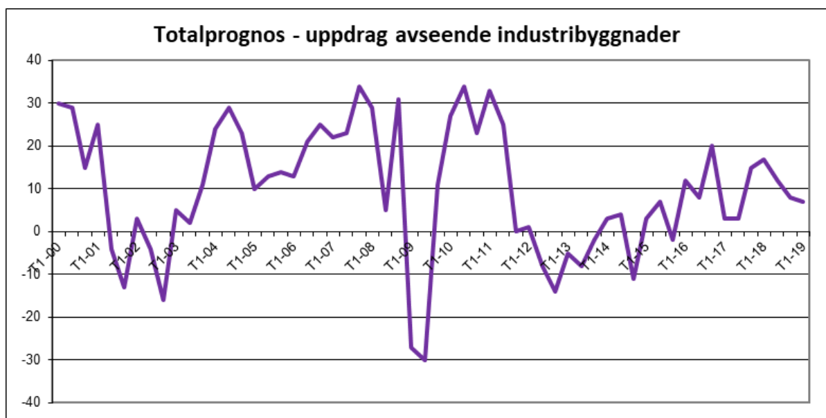
Diagram 8: Arkitekternas och teknikonsulternas sammantagna förväntningar på uppdrag avseende industribyggnader om sex månader.
