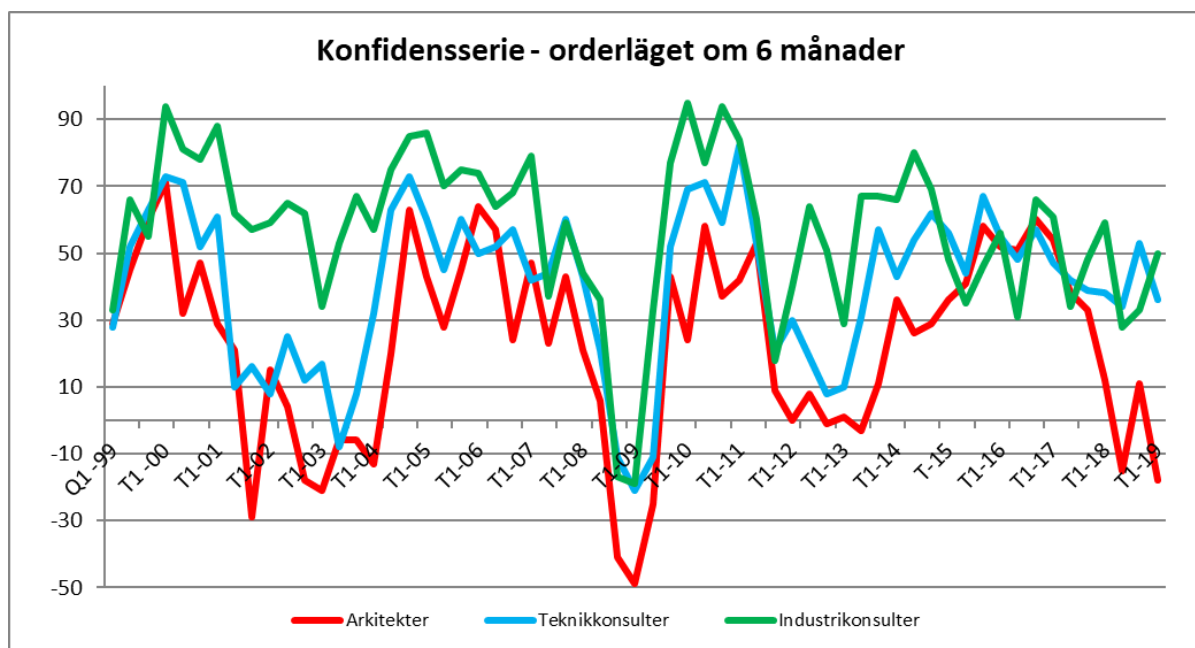
Diagram 3: Konfidensserie, förväntningar på orderläget om sex månader.
