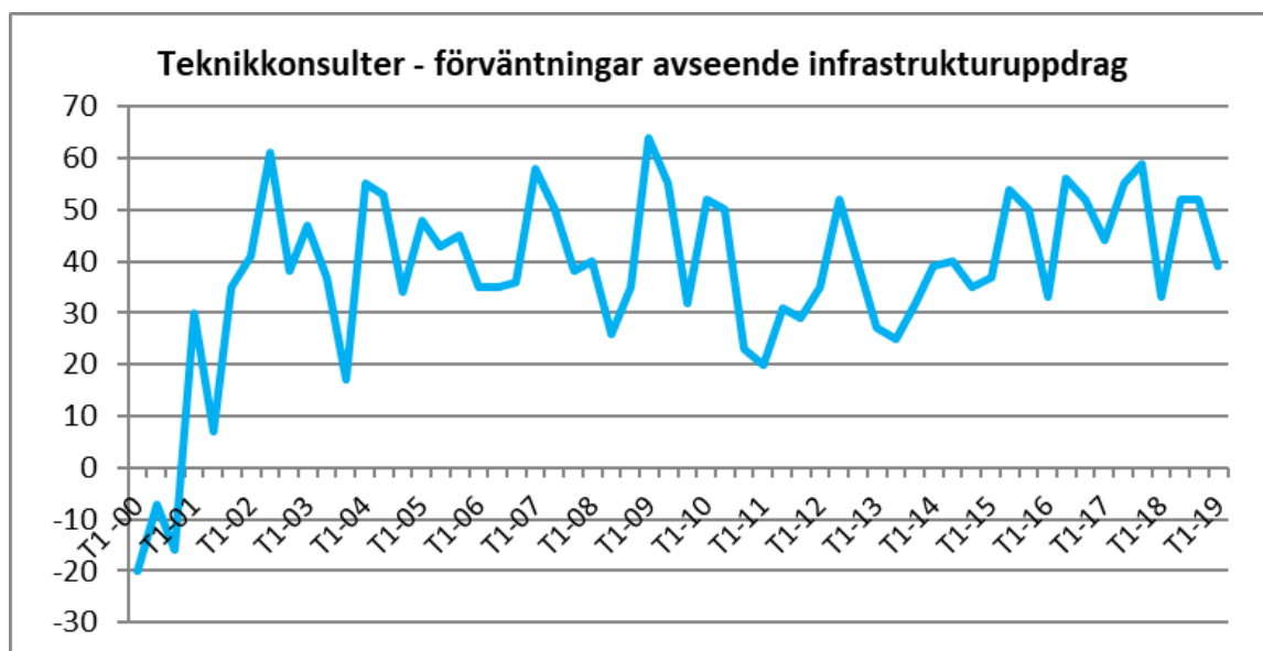
Diagram 10: Teknikkonsulternas förväntningar avseende infrastruktur om sex månader.
