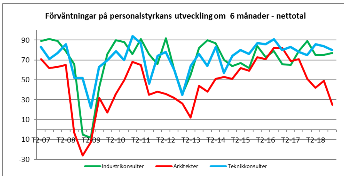
Diagram 18: Förväntningar på personalstyrkans utveckling om sex månader. Teknikksulter, arkitekter var för sig samt industriteknikkonsulter.
