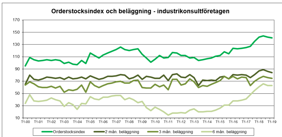
Diagram 12: Industrikonsumterna, orderstock och beläggning (två, tre och sex månader)
