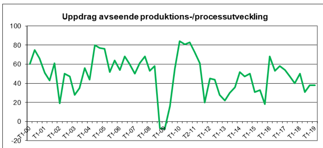
Diagram 13: Industrikonsulternas förväntningar på orderstockens utveckling för uppdrag avseende produktions- och processutveckling. Netttotal.
