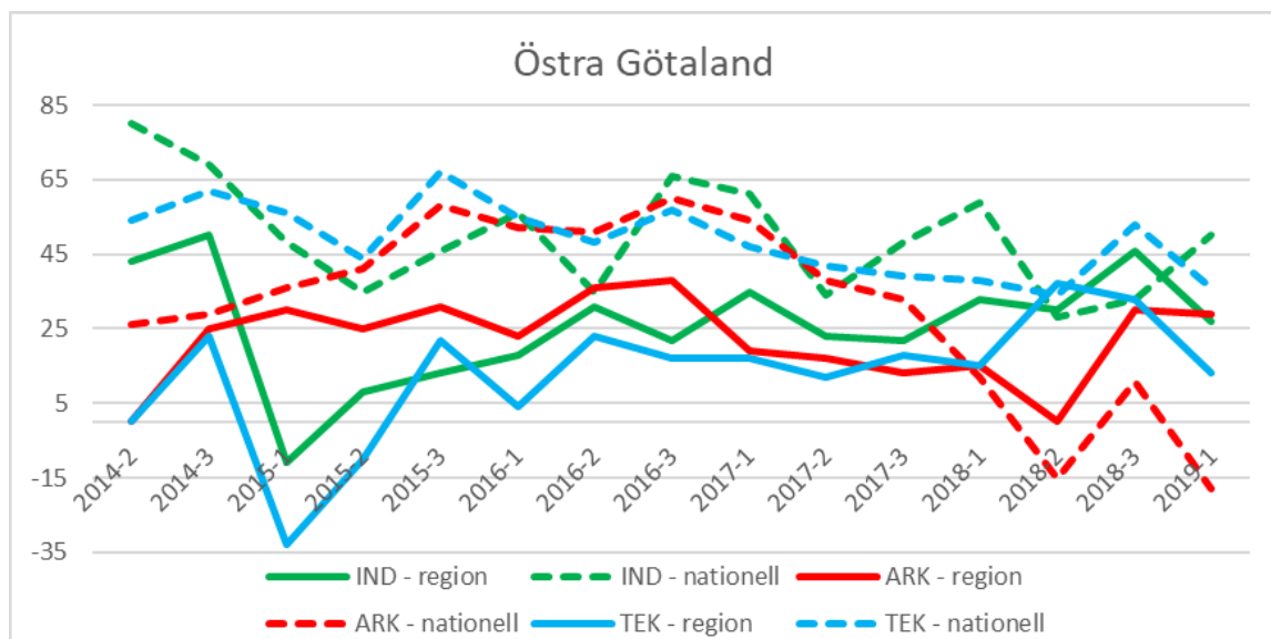
Diagram 26: Förväntningar på orderlägets utveckling i regionen (heldrager) jämfört med riket (streckat), per verksamhetsområde.
