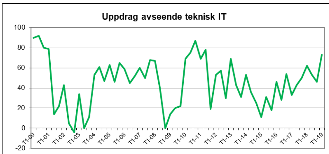
Diagram 15: Industrikonstulernas förväntningar på orderstockens utveckling för uppdrag avseende teknisk IT. Netttotal.
