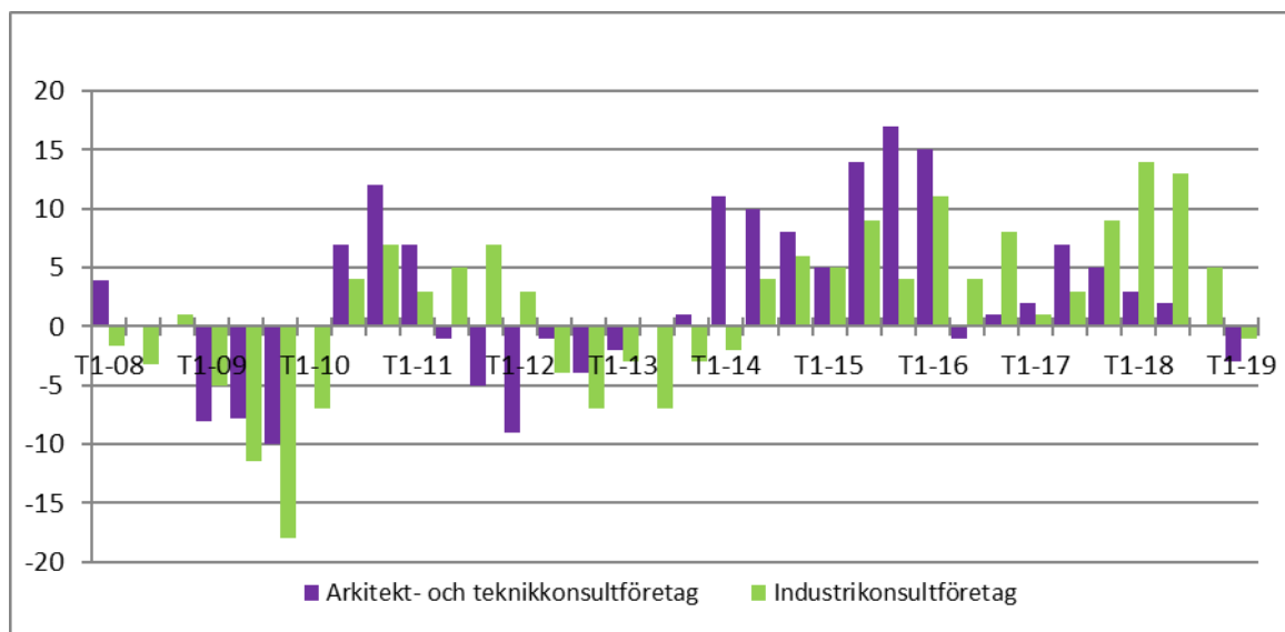
Diagram 2: Orderstocksutveckling för arkitekt- och teknikonsultföretag respektive industriksultföretag. Avser förändring av orderstocksindex i procent jämfört med samma period förra året.
