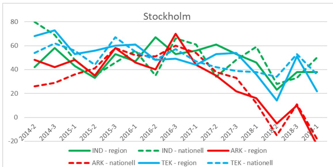
Diagram 23: Förväntningar på orderläget i regionen (heldraget) jämfört med riket (streckat), per verksamhetsområde.
