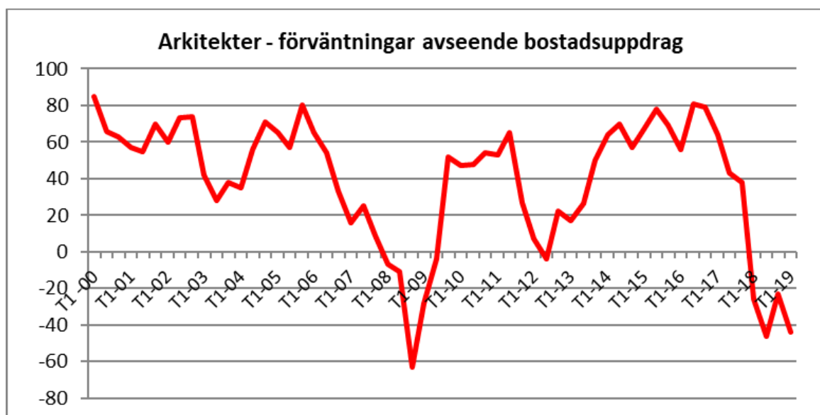
Diagram 8: Arkitekternas förväntningar avseende bostadsprojektering om sex månader.
