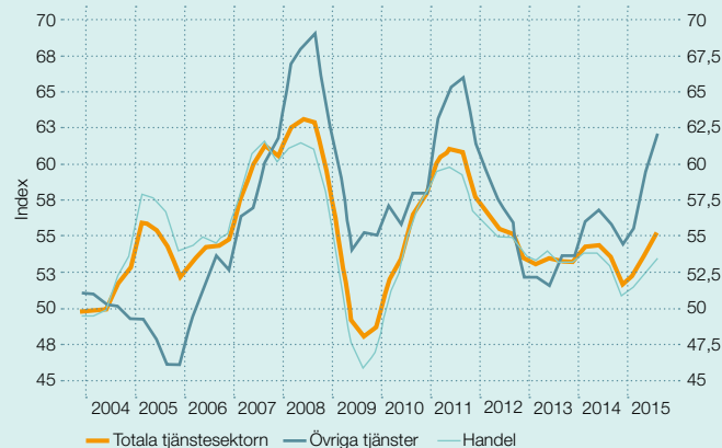
ALMEGAS PRISINDIKATOR
