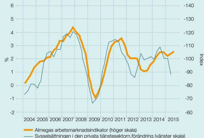
ALMEGAS ARBETSMARKNADSINDIKATOR
